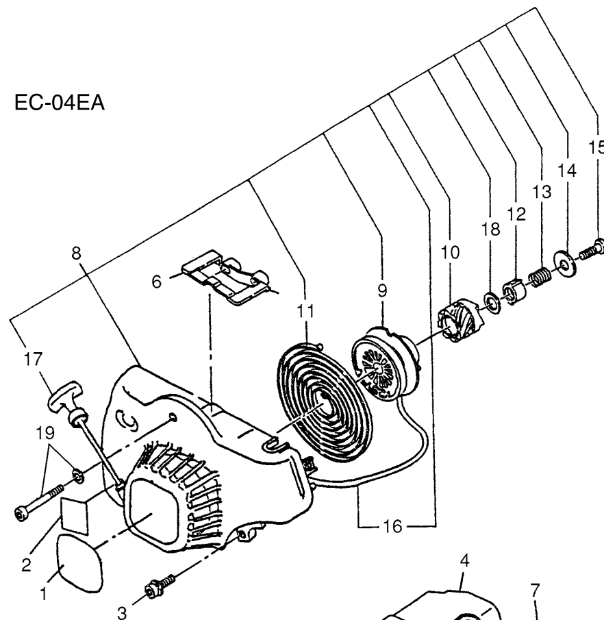
Fig.4 リコイルスタータ
